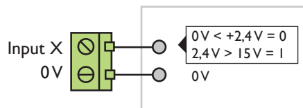
Fig. 3: Digitala ingångar
