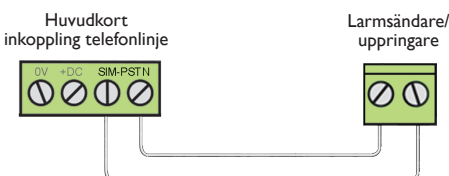
Fig. 1: Telefonuppkoppling
