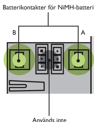
Fig. 13: Batterikontakter
