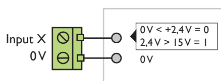
Fig. 7: Digitala ingångar
