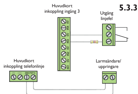
Fig. 3: Sabotageskydd för telefonlinje
