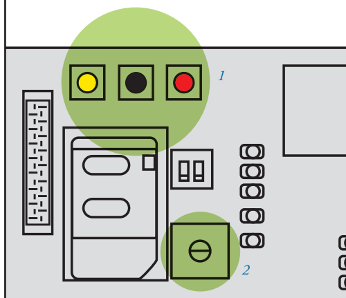
Fig. 15 Knappar (1) och positionsbrytare (2)
