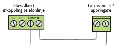
Fig. 1: Telefonuppkoppling
