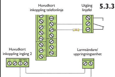
Fig. 2: Sabotageskydd för telefonlinje
