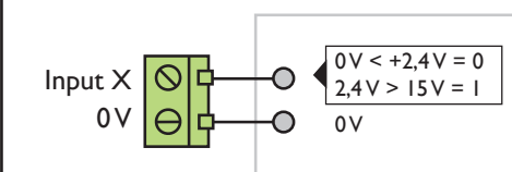
Fig. 6: Digitala ingångar
