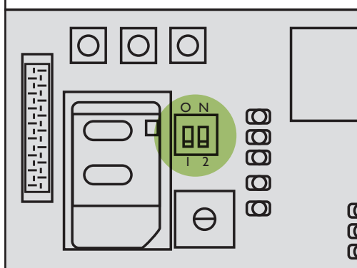
Fig. 16 DIP-omkopplare DP1 och DP2
