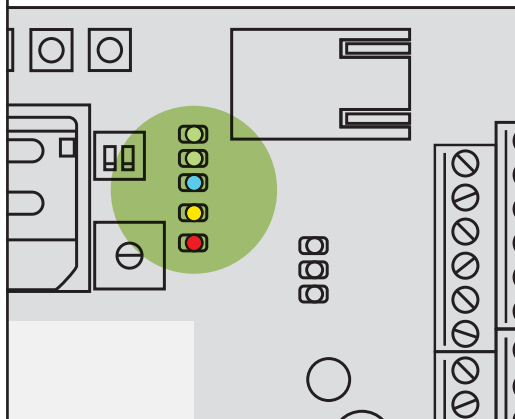
Fig. 17 LED-indikatorer
