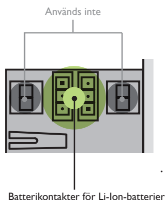
Fig. 13 Batterianslutning
